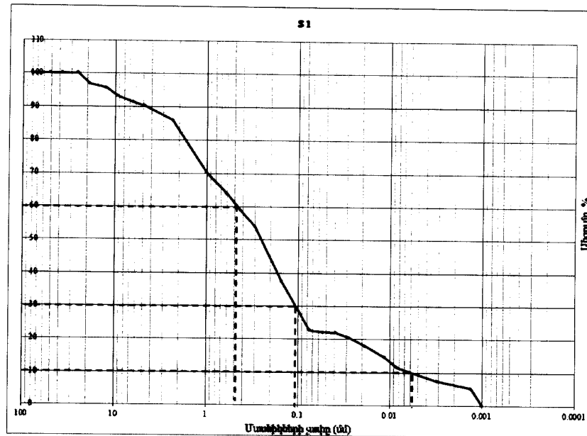
Գծապատկեր 1. Նմուշ № 1-ի հատիկաչափական կազմը
